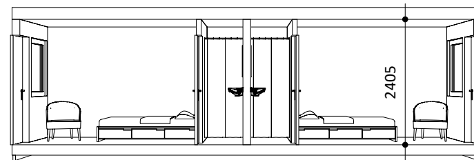
03 Sektion A-A 1:100
