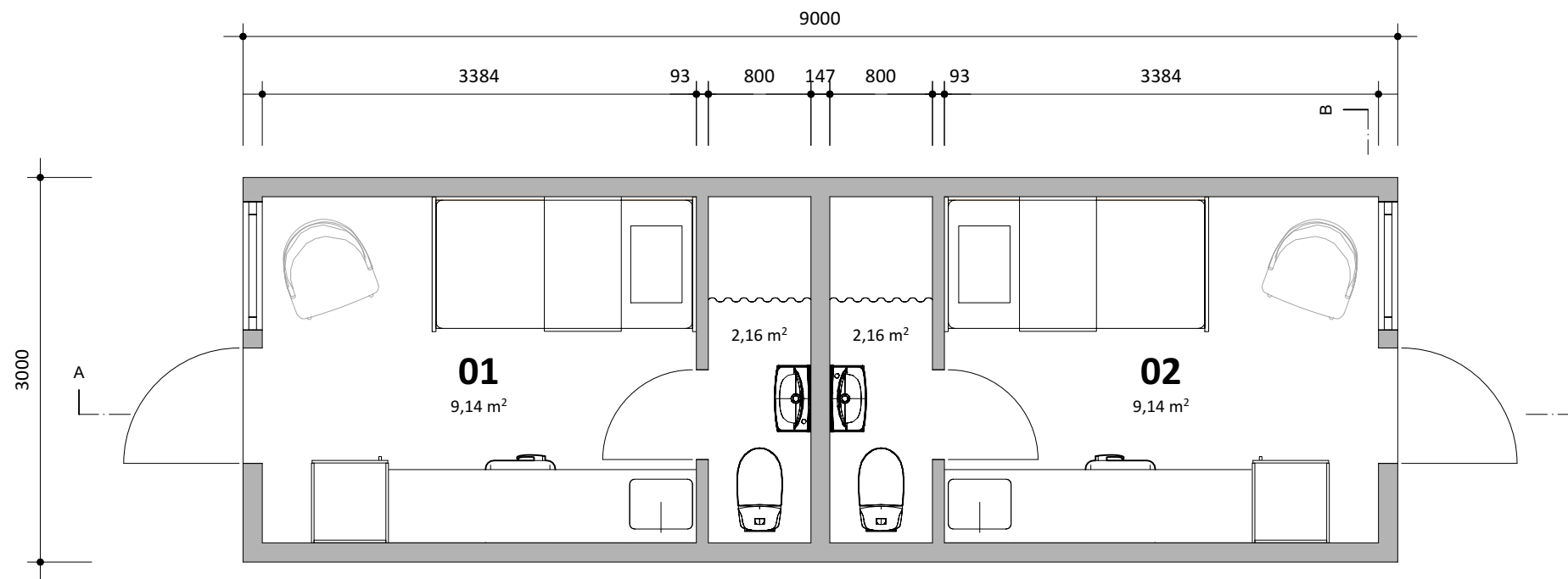
01 Planlösning 1:50
